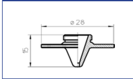
Dysor HD.
